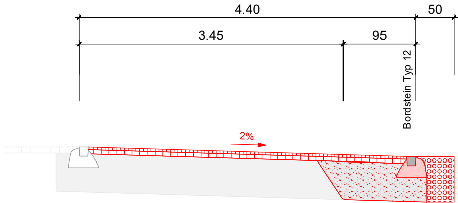
Normalprofil 1
