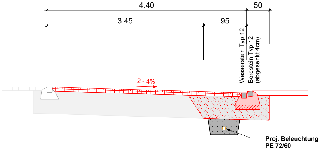
Oberbau Fahrbahn:
